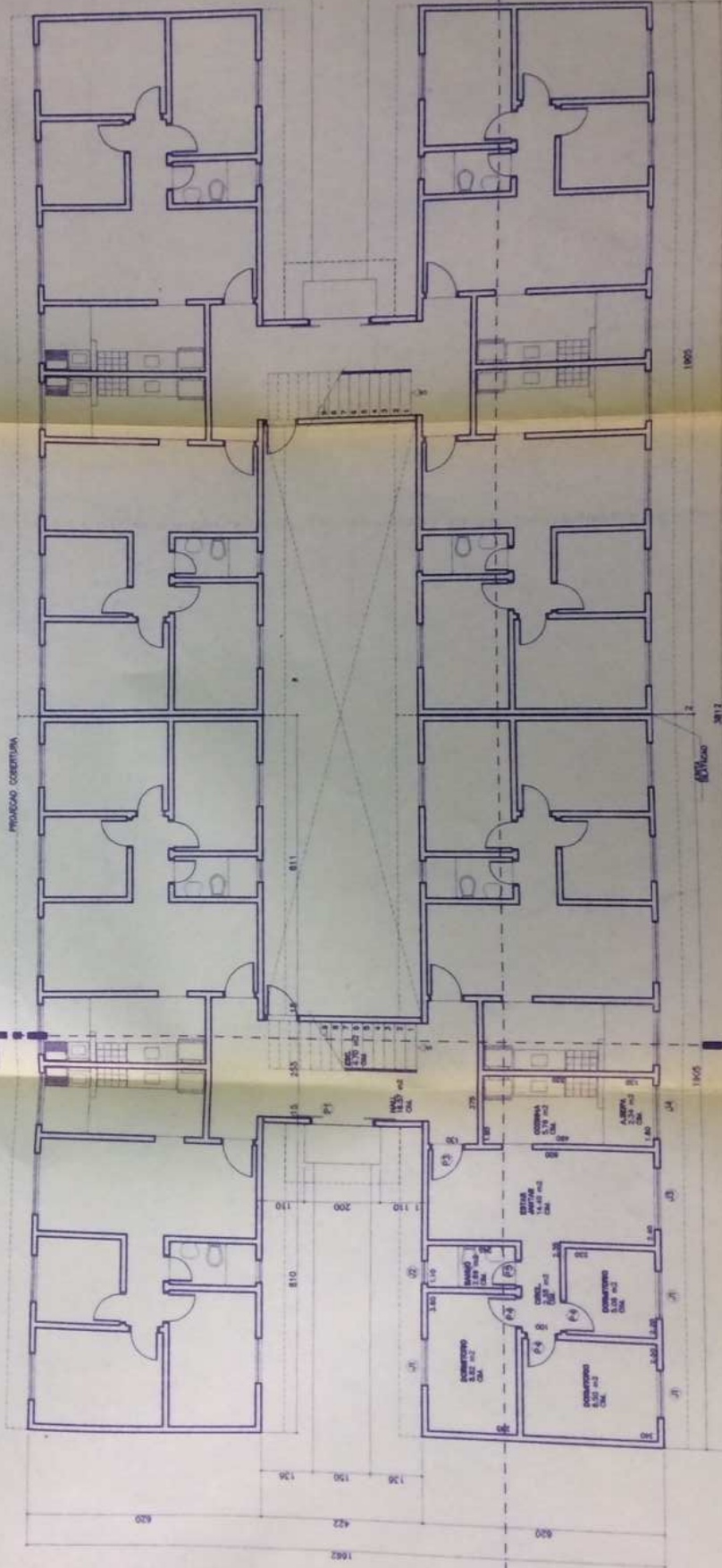
BLOCCO PAV. TERREO (TIPO 3 DORMITORI) ESQ. 1:100
